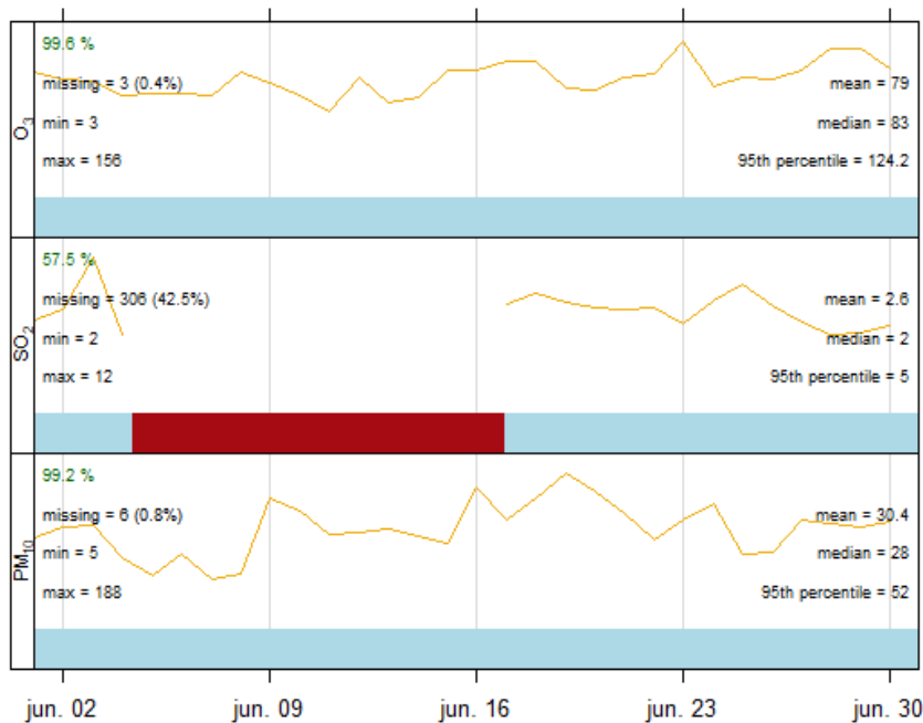
Estación de Illescas - Evolución mensual, Junio de 2025
